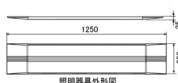
照明器具外形図
